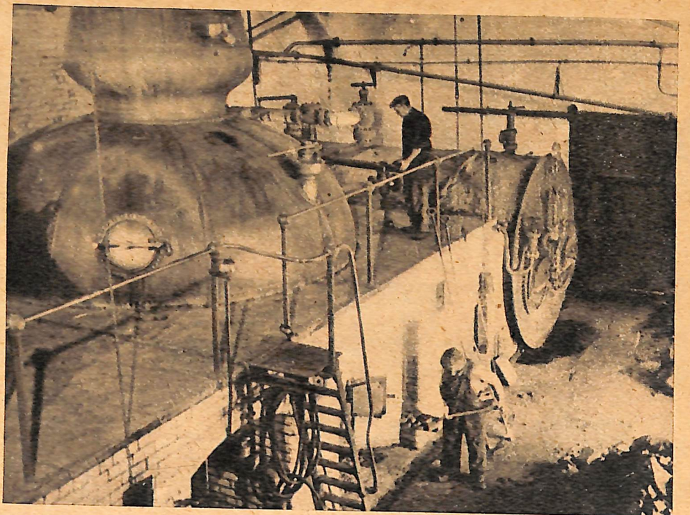
Starczyłoby na ugoszczenie dywizji... Miedziana retorta, w której odbywa się proces destylacyjny
