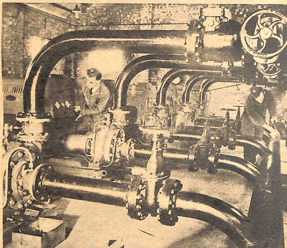
Pompy elektryczne tłoczą do rur paliwo
