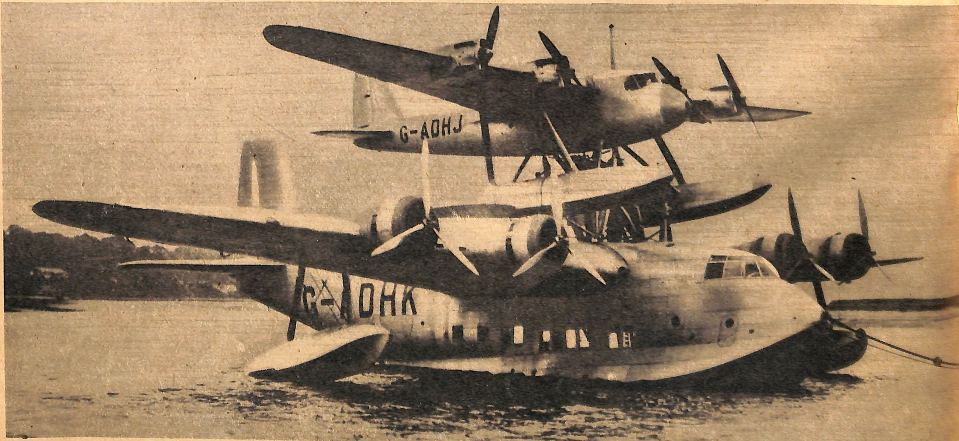
Ten dziwnie wyglądający samolot konstrukcji brytyjskiej, złożony z dwóch aparatów, rozłączających się w czasie lotu, używany był w Anglii dla celów doświadczalnych. Doświadczenie to przydało się jego konstruktorom w późniejszej produkcji dobrze znanych bombowców typu „Stirling” oraz wodnopłotowca „Short Sunderland”
